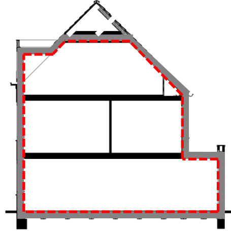
Figuur 2b: Te meten zone valt binnen de thermische schil (= luchtdichte schil); de vloering ligt buiten de thermische schil ; vliozoluken/knieschotten behoren tijdens de meting gesloten te zijn – zie hiervoor paragraaf 5.1.5.
