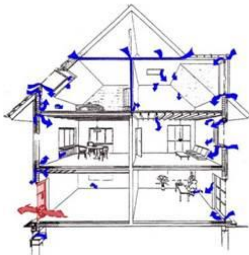
Figuur 2c: voorbeeld van veelvoorkomende infiltratie (bron: BlowerDoor GmbH)
