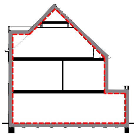
Figuur 2a: Te meten zone valt binnen de thermische schil (= luchtdichte schil); ook de vloering ligt binnen de thermische schil ; vliozoluken behoren tijdens de meting open te zijn; knieschotten behoren tijdens de meting gesloten te zijn – zie hiervoor paragraaf 5.1.5.
